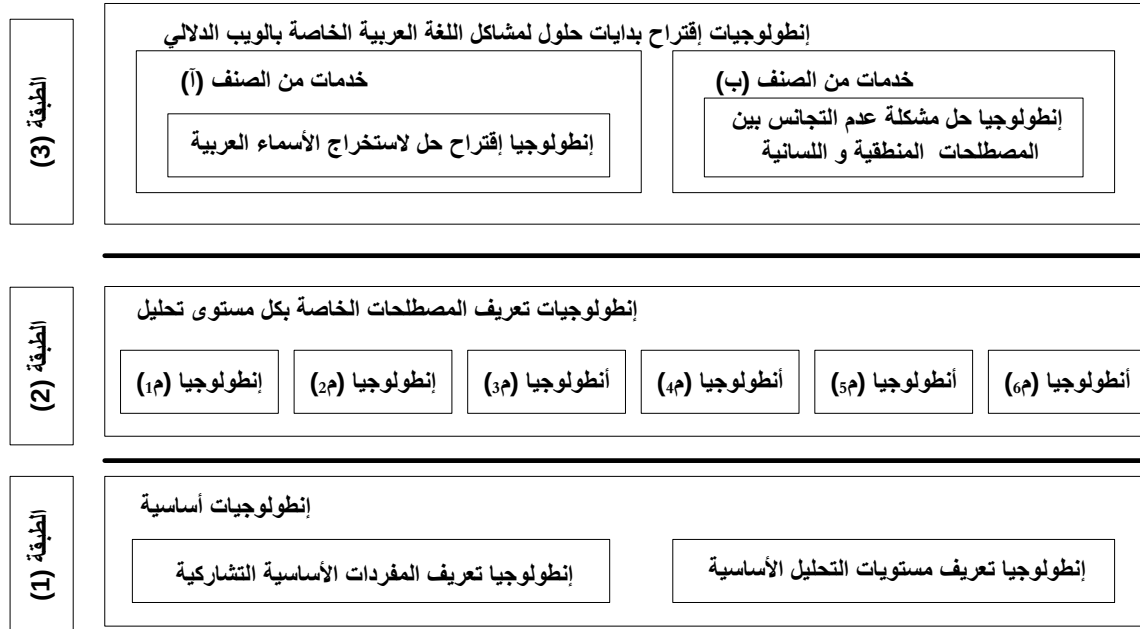
الشكل (9) الإنطولوجيات المساعدة موزعة على الطبقات الثلاثة
