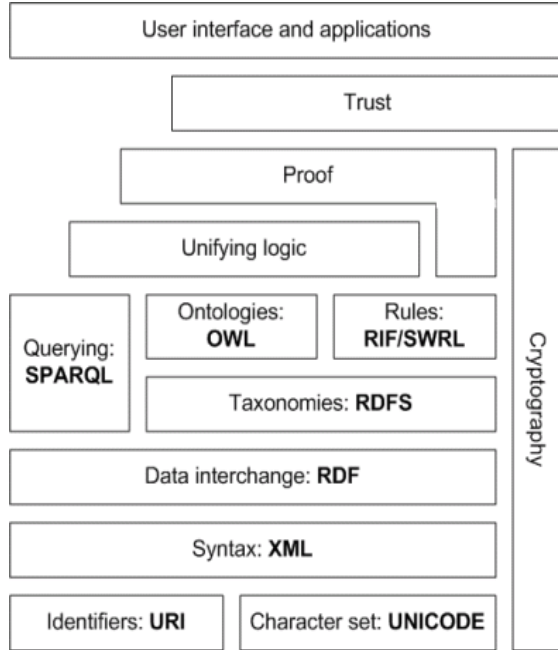
الشكل (1) طبقات الويب الدلالي [20]
